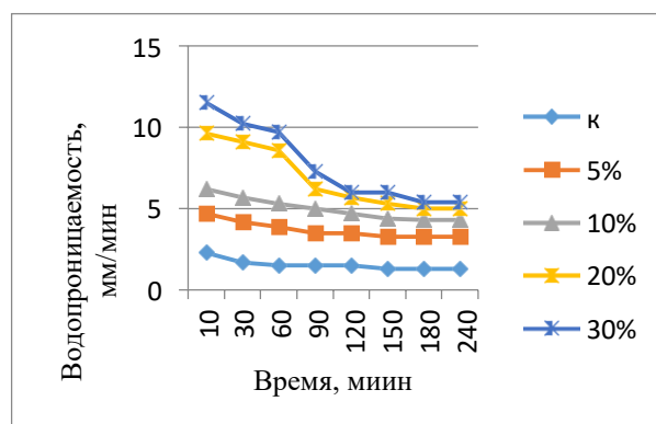
Рисунок 2. Водопроницаемость образцов почвы в зависимости от дозы вносимого биоугля.
