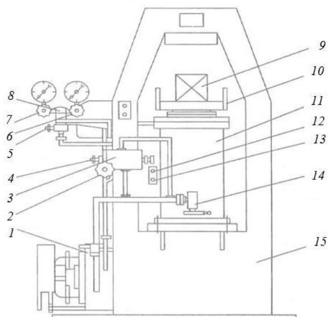
Рис. 4. Схема гидравлического пресса БКК-200:
