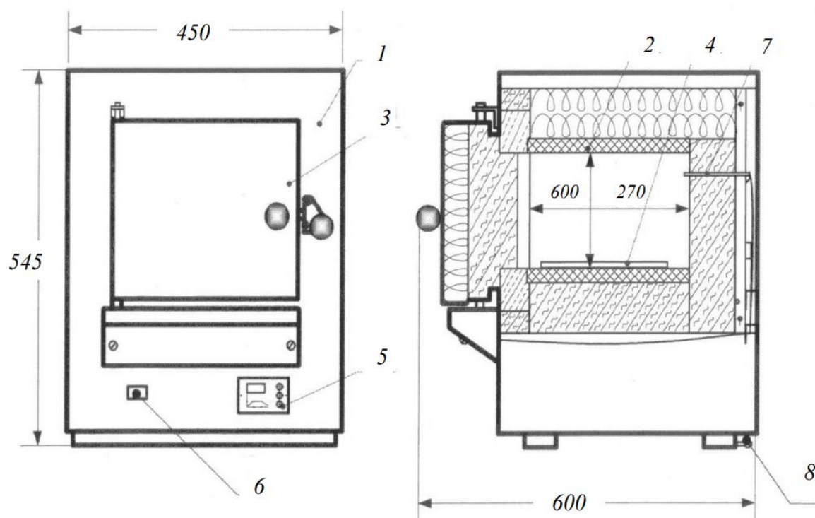
Рис. 1. Камера электропечи СНОЛ 6/10
